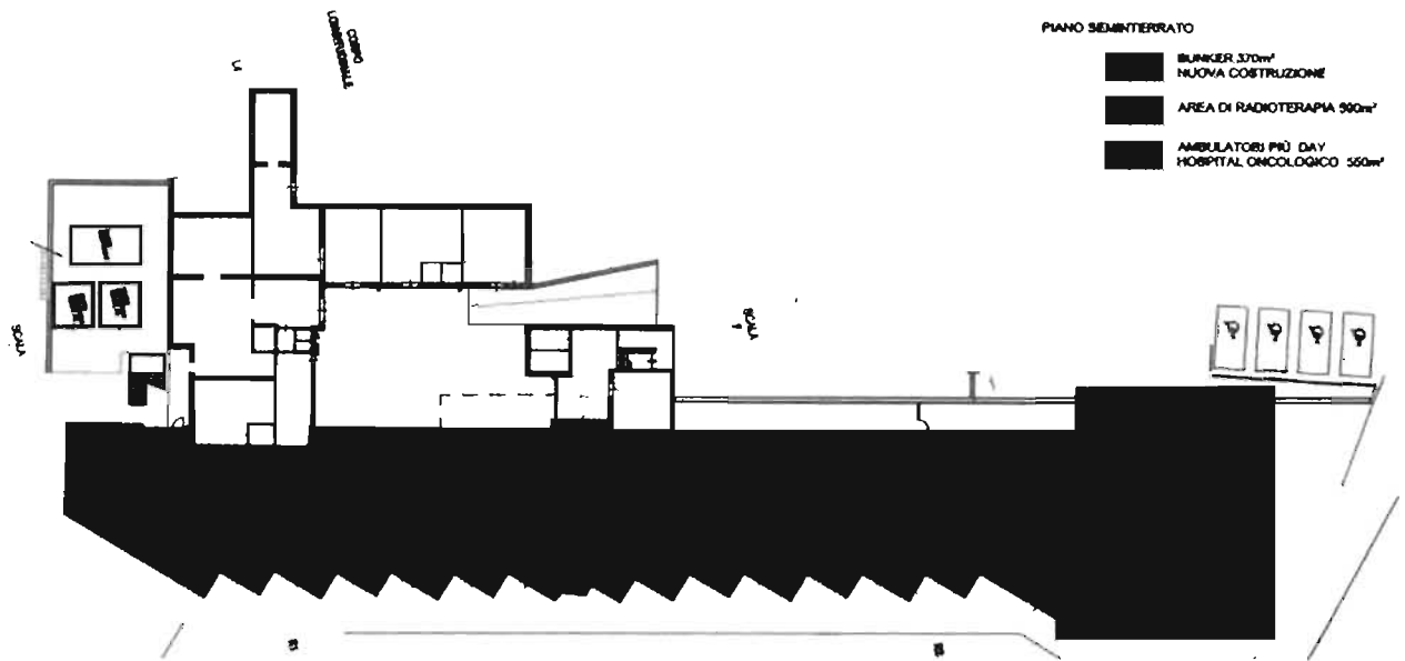
Figura 8 – Piano Semicinterrato Reparto di Radioterapia identificazione delle tre attività
